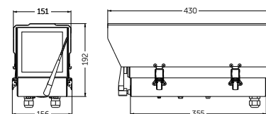
MITRE 901 / 801
