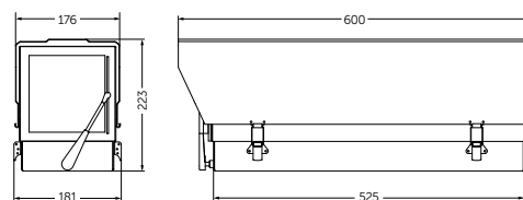
MITRE 900 / 800
