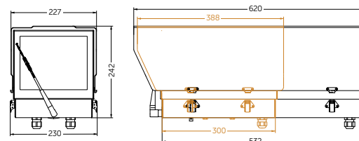
MITRE 903 / 903 SHORT
